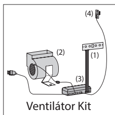
Ventilátor Kit (bekötés után is szerelhető, a burkolás előtt) alkotóelemei: szinoptikus panel (1), ventilátor (2), szabályozó (3), érzékelő(4)
